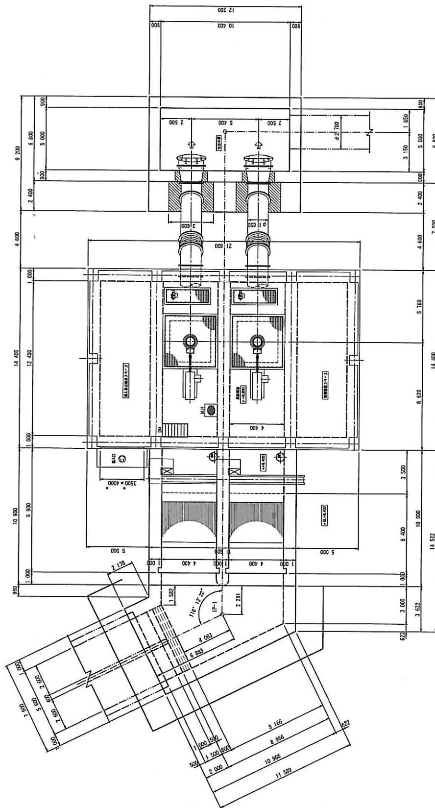
平面図 S = 1 : 100
