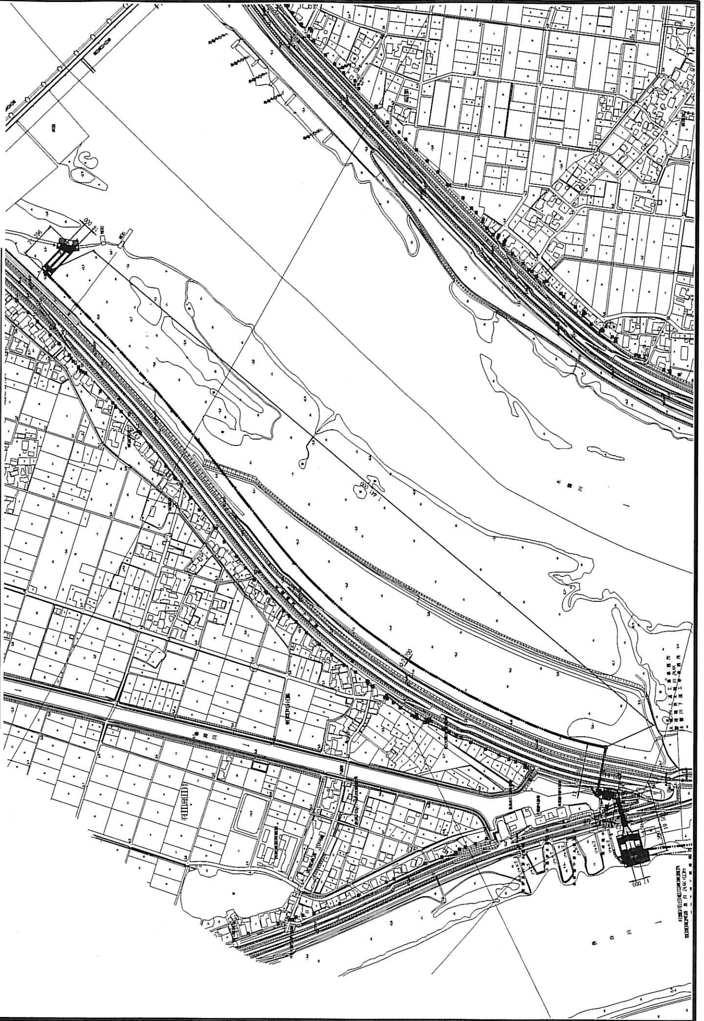
木曾川導水路（最下流案）全体平面図 Q=11.52 \text{ m}^3/\text{s} S=1:2,500
